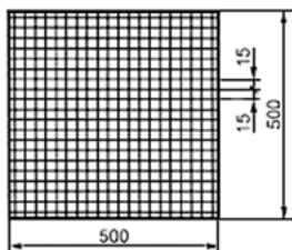
Рисунок 3 Форма рифления с квадратными рифами
